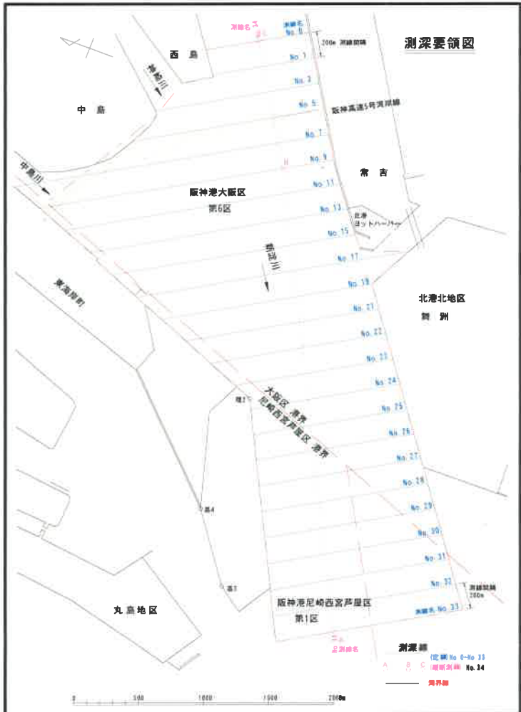
図-2 深浅要領図
